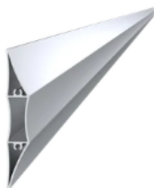
Profil 100x16mm, L-6000mm, hliník bez povrchovej úpravy
