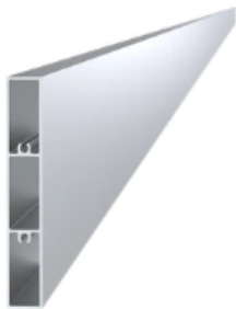
Profil 100x16x6000mm, L-6000mm, hliník bez povrchovej úpravy
